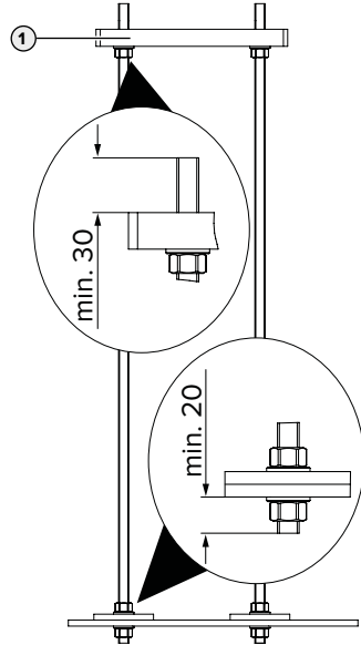
Afb. 2: Positie van de ringen en moeren [mm]
