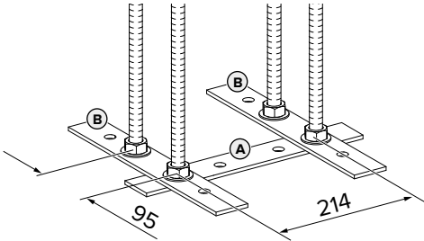
Afb. 1: Afmetingen [mm]
