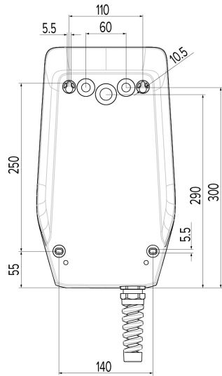
Fig. 6: Bormått [mm]
