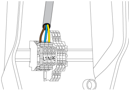
Afb. 7: Aansluiting voedingspanning
