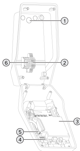
Fig. 4: Vy inifrån
