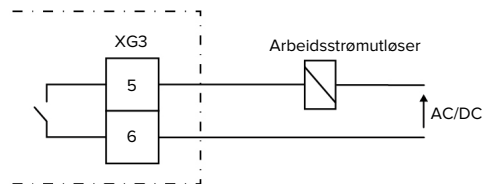
Fig. 8: Prinsipielt koblingsskjema: tilkobling av ekstern arbeidsstrømutløser
