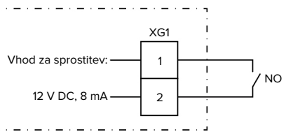
sl. 12: Osnovna vezalna shema: priključitev zunanega preklopnega kontakta
