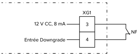
Fig. 11 : Schéma de principe : raccordement d'un contact de commutation externe
