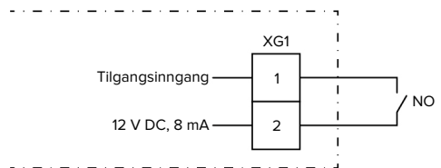
Fig. 12: Prinsipielt koblingskjema: tilkobling av en ekstern bryterkontakt
