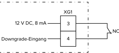
Abb. 11: Prinzipschaltbild: Anschluss eines externen Schaltkontakts
