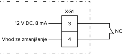
sl. 11: Osnovna vezalna shema: priključitev zunanega preklopnega kontakta
