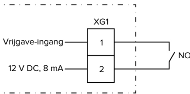
Afb. 12: Principeschema: Aansluiting van een extern schakelcontact
