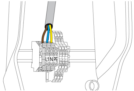
Fig. 7: Tilkobling spenningstilførsel
