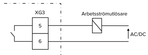
Fig. 8: Principkopplingschema: anslutning av extern arbetsströmutlösare
