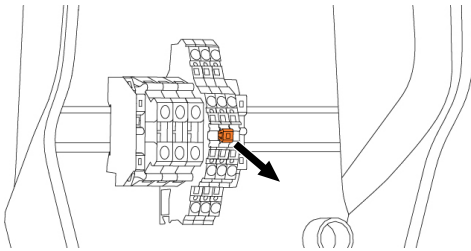
Рис. 10: Извлечение перемычки
