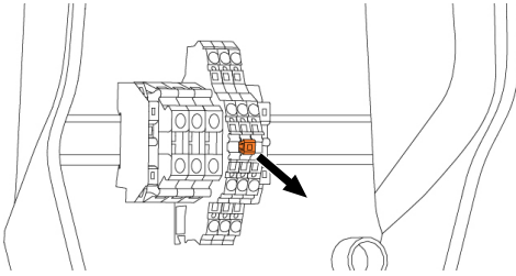
Abb. 10: Brücke herausnehmen
