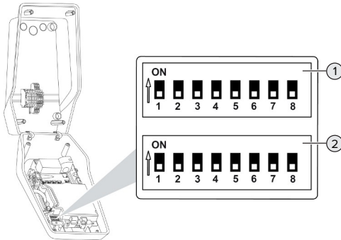
Fig. 9: DIP-brytare (leveranstillstånd)
