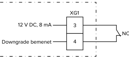
11. ábra: Elvi kapcsolási rajz: külső kapcsolóérintkező csatlakoztatása
