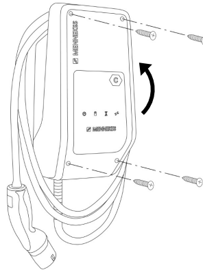
Fig. 14: Stänga produkten
