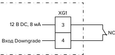
Рис. 11: Принципиальная схема: подключение внешнего переключающего контакта
