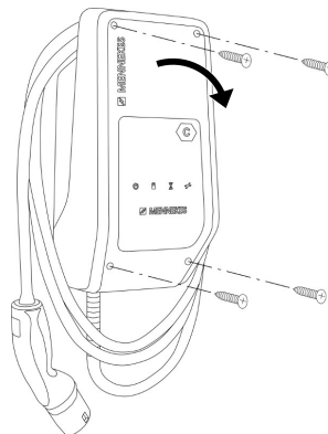
Fig. 5: Öppna produkten
