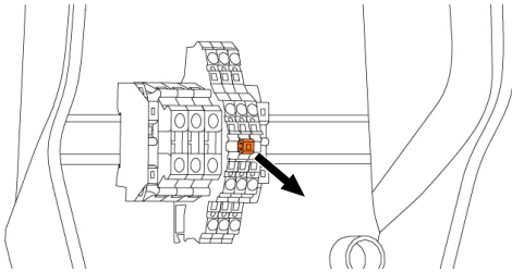
Afb. 10: Brug uitnemen
