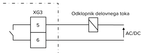
sl. 8: Osnovna vezalna shema: priključitev zunanje odklopnika delovnega toka
