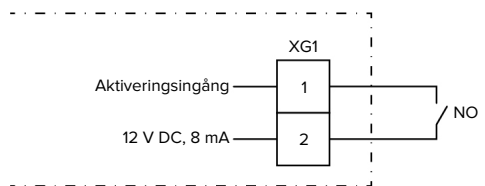
Fig. 12: Principkopplingschema: anslutning av en extern brytarkontakt
