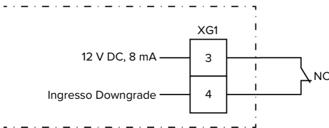
Fig. 11: Diagramma unifilare: collegamento di un contatto di commutazione esterno
