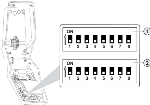
Afb. 9: Dipschakelaar (uitleveringstoestand)
