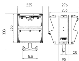
Disegno 1 MB 630
