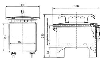
Disegno 5 MB 43 Dim. in mm
